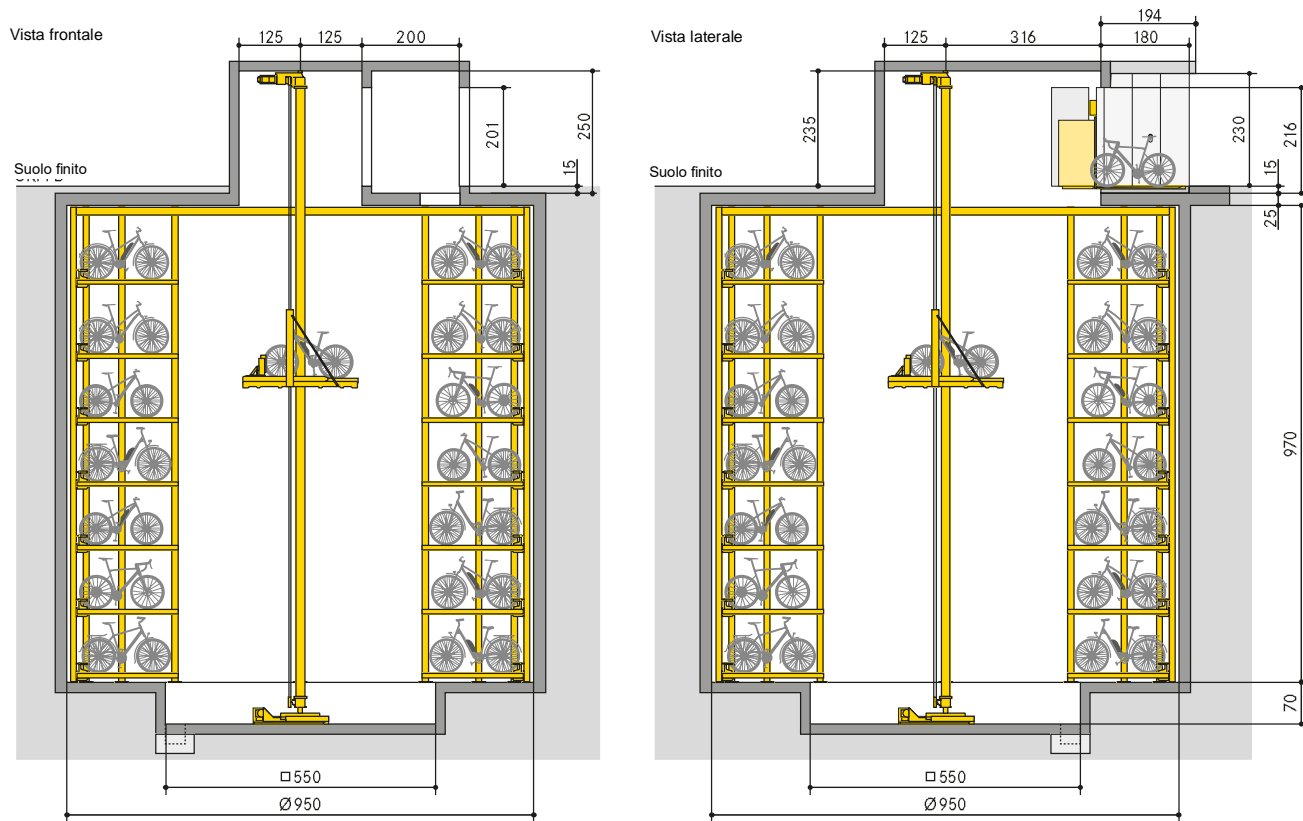
Sezione livello di parcheggio
